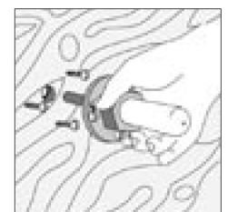
Leichtes Abnehmen durch Bajonett- verschluß
